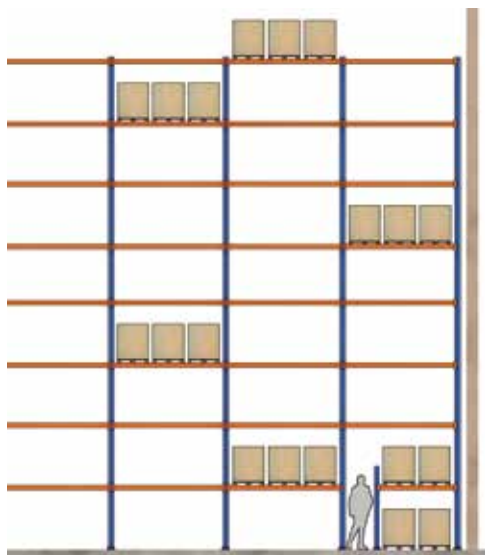
Vue en élévation d'une installation avec passage
