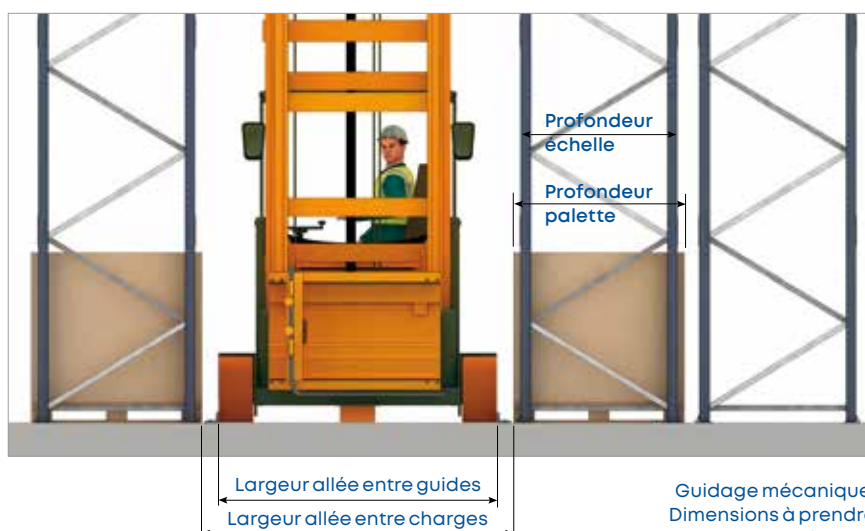
Guidage mécanique. Schéma général
